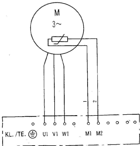
图 4 带 PTC 元件电机接线图
