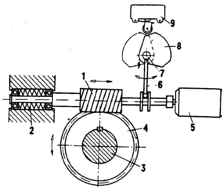
图 1 电动执行机构工作原理
