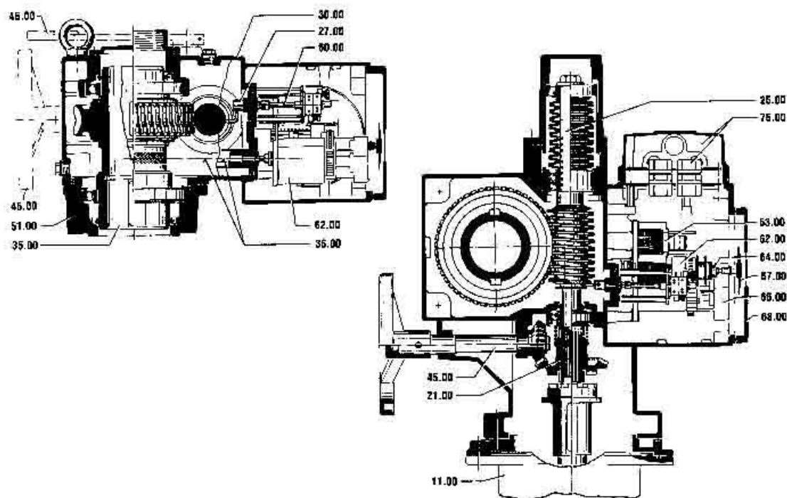
图 2-b 2SA3.3~2SA3.4 电动执行机构结构
