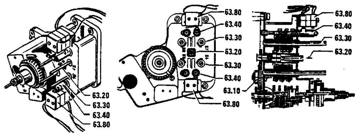
图 10 行程控制计数器机构 RSW
