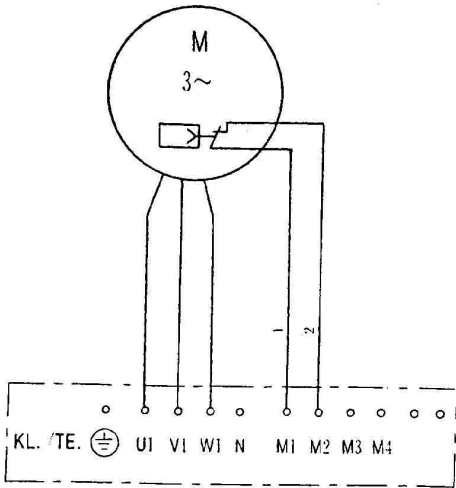
图 3 带热控开关电机接线图
